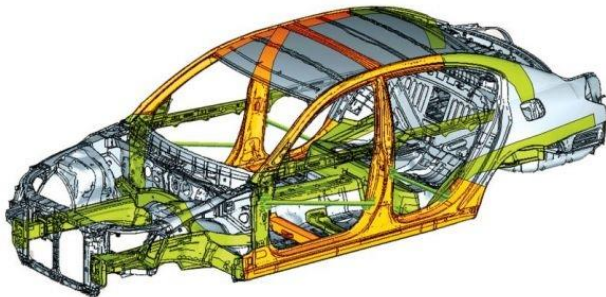
[그림1] 구형 제네시스의 18% UHSS 적용(노랑색)
